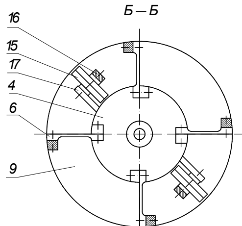
Рис. 2. Схема розташування пружин та пневмодемпферів
